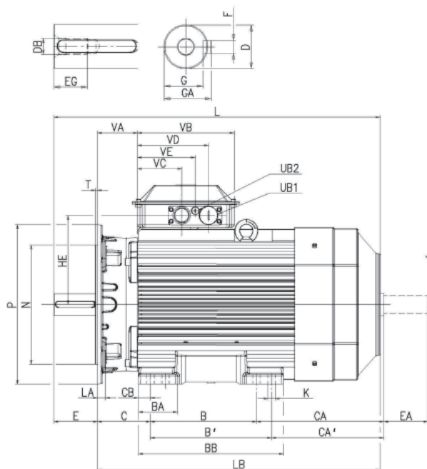
Foot- and flange-mounted motor; IM B35 (IM 2001), IM 2002
