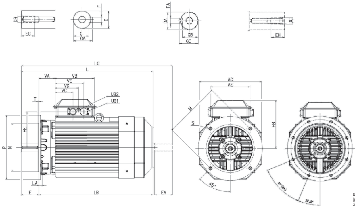
Flange-mounted motor; IM B5 (IM 3001), IM 3002
