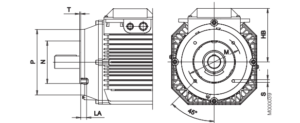
Flange-mounted motor, small flange; IM B 14 (IM 3601), IM 3602
